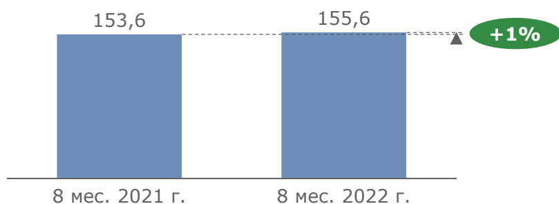
ПРОИЗВОДСТВО СЕЛЬСКОХОЗЯЙСТВЕННОЙ ТЕХНИКИ, млрд руб. (с НДС)
